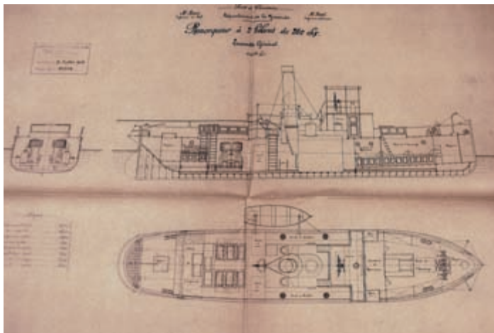
Plan d'un remorqueur à deux hélices construit aux Chantiers navals de Barriol
